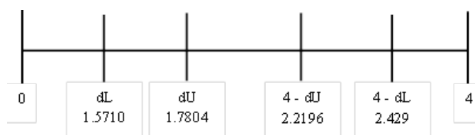
Gambar 3. Mapping Autokorelasi
